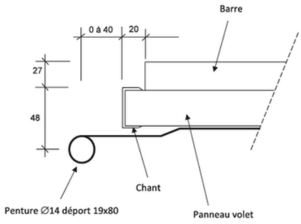
Sans feuillure Pose en tunnel ou en applique
