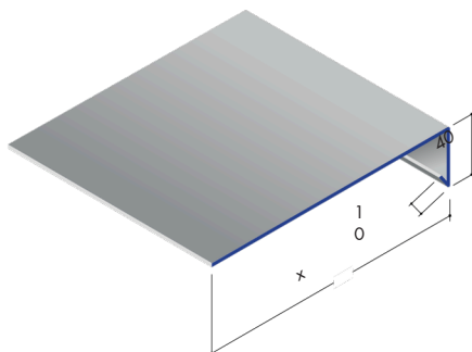
Bardage de façade
