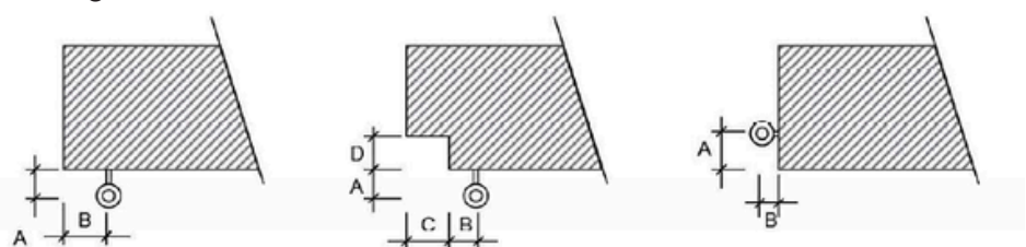
Sans feuillure Pose en tunnel ou en applique
