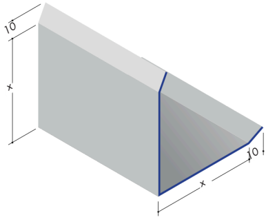
Bande d'égouts
